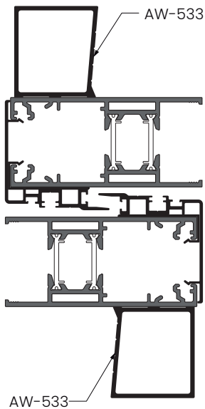
Abertura con refuerzo doble
