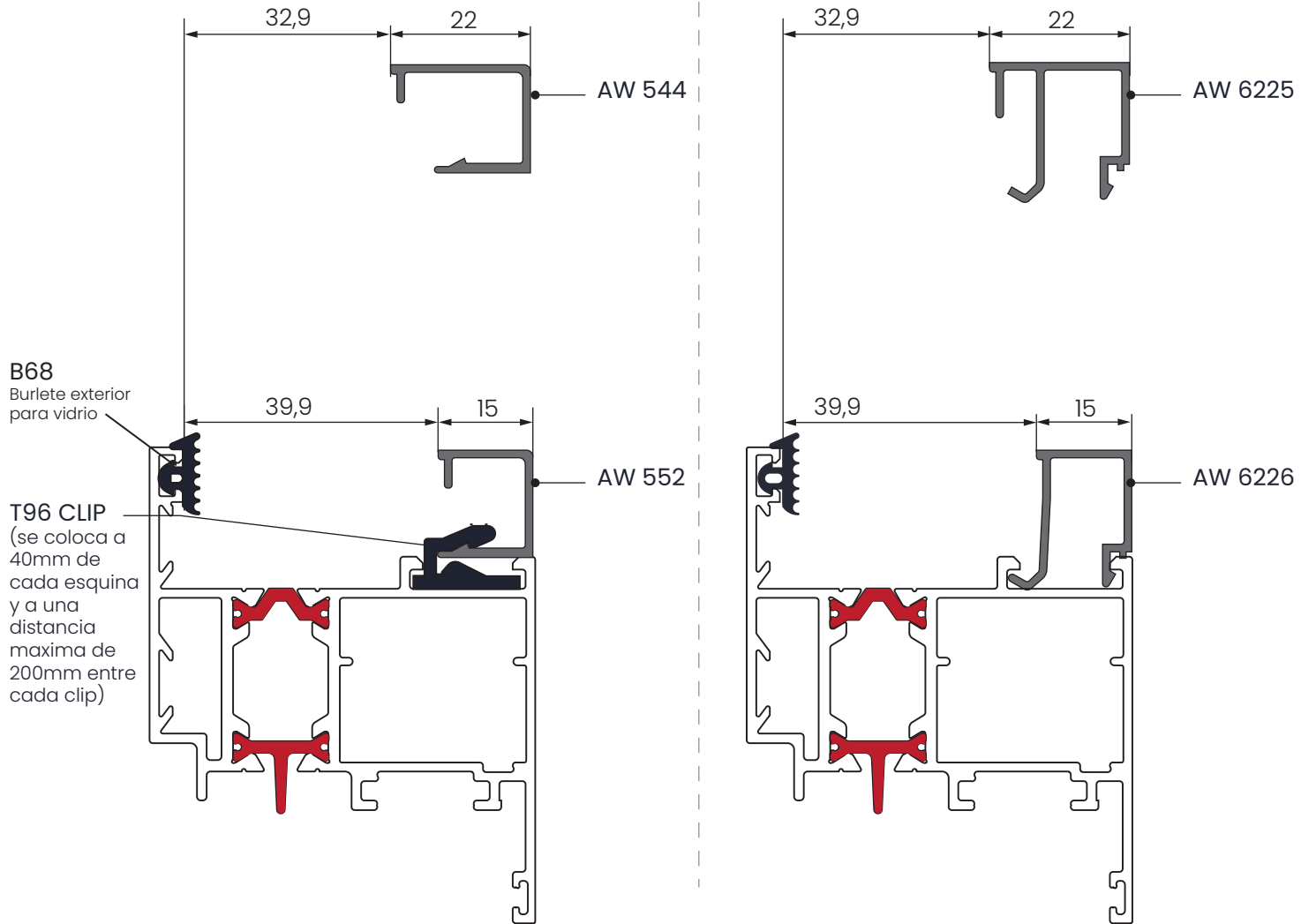
CONTRAVIDRIOS CORTE A 45°
